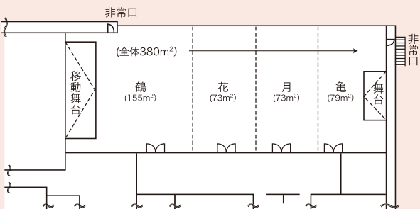
2F (2階の平面図の一部)
